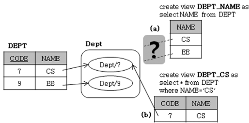
그림 5 뷰와 클래스
