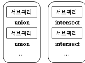
그림 7 뷰의 형태
