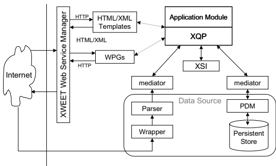
그림 5 XWEET 구조
