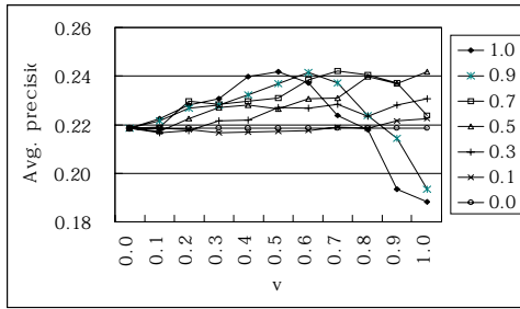
그림 10 f에 따른 v값의 변화
