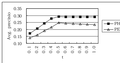
그림 9 t변화 그래프
