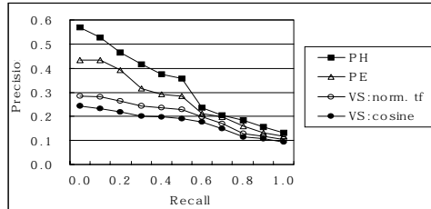
그림 7 모델별 정확률-재현율 그래프
