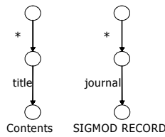
그림 3 SRP 질의 예
