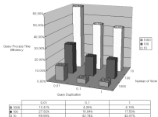
그림 12 질의의 중복성에 따른 응답시간
