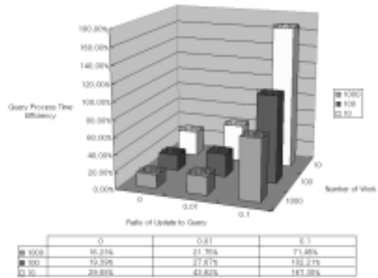
그림 11 하나의 질의에 대한 지역 편중성이 없을 때의 응답시간
