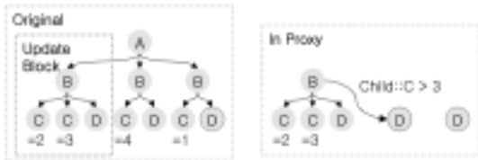
그림 9 갱신블록(Update Block)내의 노드만을 추가로 기록
