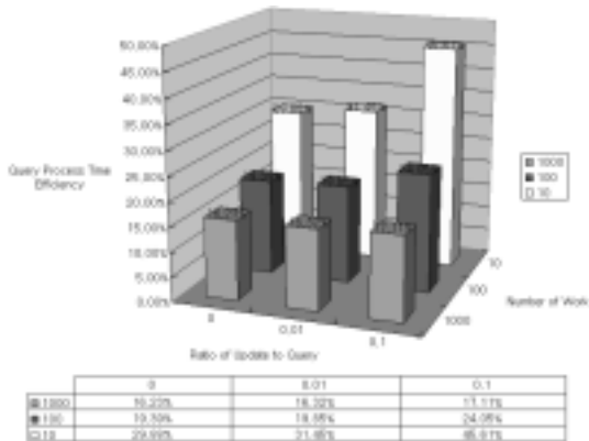
그림 10 하나의 질의에 대한 지역 편중성이 심할 때의 응답시간
