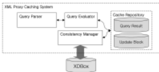
그림 5 XML 프록시 캐쉬 시스템 구조
